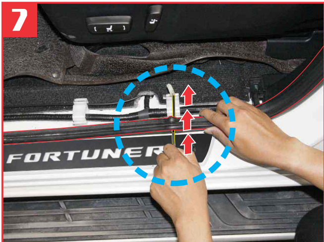
The correct position to mounting scuff plate with LED after marking position with crayon. แสดงตำแหน่งติดตั้งชายบันไดเรืองแสง
