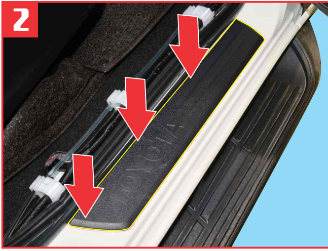
Attached original scuff plate ( the short one ) by organizing in correct position as shown. นำแผ่นปิดชายบันได(ชิ้นเล็ก)ที่ถอดไว้ ประกอบเข้าตำแหน่งเดิม เพื่อกำหนดตำแหน่งการติดตั้งชายบันไดเรืองแสง
