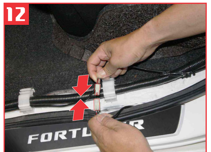
Connect the power cord into the socket of the Lamp เชื่อมต่อขั้วปลั๊กของชายบันไดเรืองแสง เข้ากับ ขั้วปลั๊กของชุดสายไฟชายบันไดเรืองแสง
