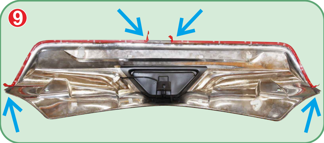
PULL THE DOUBLE SIDED TAPE OFF THE LITTLE AS PHOTO SHOWN. ลอกเทปกาวที่บริเวณขอบของแผงกันกระแทกฯ ออกเพียงเล็กน้อย
