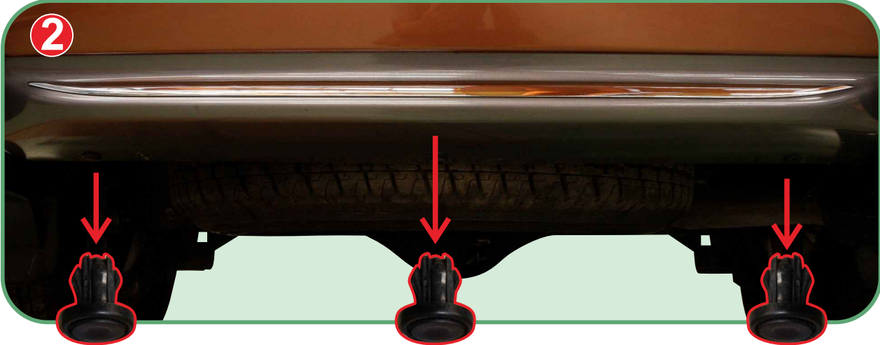
REMOVE THE GROMMET BELOW THE 3 POINTS OUT. ถอดคลิปล็อกพลาสติกด้านล่างกันชนหลังทั้ง 3 จุด
