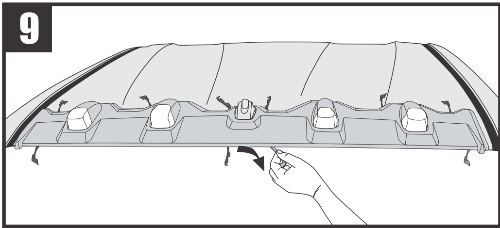
Peel off the rest of double sided tape as shown. ลอกเทปกาวออกให้หมด
