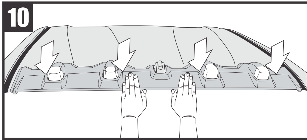
Press it firmly กดไฟแอลอีดีหลังคาให้แน่นสนิทกับตัวรถยนต์ ดังภาพ
