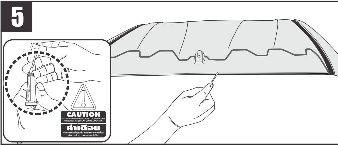
***PLEASE NOTE! IMPORTANT PROCESS!*** Apply primer (provided) on marking position before installing for better adhesion. ทาน้ำยา พายเมอริ์ ด้านในของรอยดินสอเทียน เพื่อการยึดเกาะของเทปกาว 3M เต็มประสิทธิภาพ
