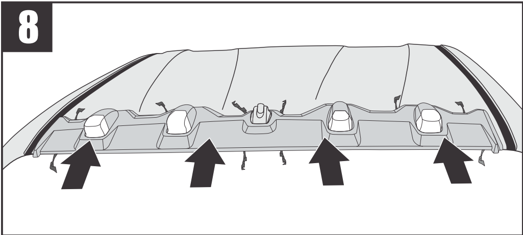
Press it firmly ติดตั้งไฟแก็ปหลังคาเข้ากับรถยนต์
