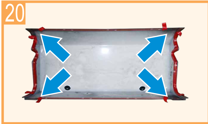
Peel off double-sided tapes on base plate (provided) a bit as shown ลอกเทปกาฐานรองป้ายทะเบียนออกบางส่วน ตามภาพ
