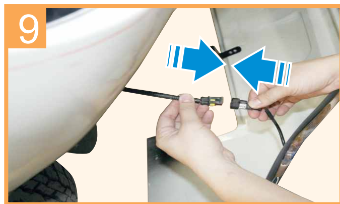
Connect LED wire of rear skirt to lamp wire as shown เชื่อมต่อสายไฟเข้ากับชุดดวงไฟ LED สเกิร์ตหลัง ตามภาพ
