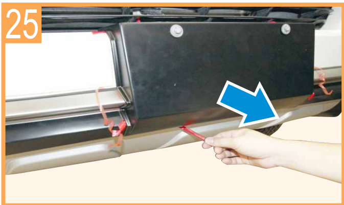
Peel off the rest of double-sided tapes on base plate as shown ลอกเทปกาฐานรองป้ายทะเบียนออก ตามภาพ
