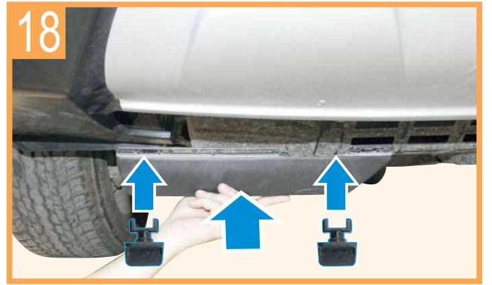
Reassemble attached plate as shown ติดตั้งแผ่นพลาสติกใต้กันชนหน้ากลับตำแหน่งเดิม ตามภาพ
