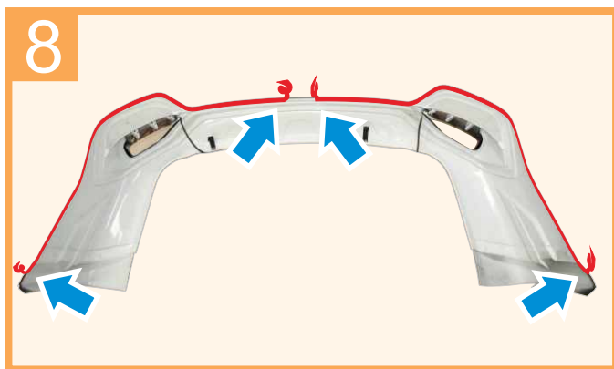
Peel off a small parts of double sided tapes on back side of rear skirt with LED as shown ลอกเทปกาวออกเพียงบางส่วน
