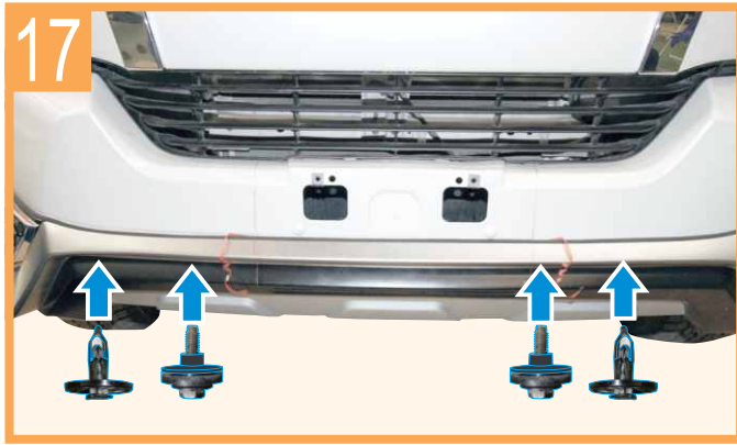
Screw (original) front skirt with DRL to car as shown ใช้สกรูยึดชุดสเกิร์ตหน้าเข้ากับตัวรถยนต์ ตามภาพ
