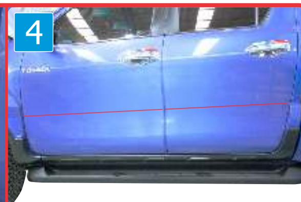
3 & 4 ) Attached rear body cladding to marking position with crayon as shown. ทาบกาบข้างประตูหลังเข้ากับตัวรถ โดยจัดวางตำแหน่งให้อยู่แนวเดียวกับ กาบข้างประตูหน้า แล้วใช้ดินสอเขียนขีดเส้น เพื่อกำหนดตำแหน่งทาบท้ายรองพื้น(3M) ดังภาพ
