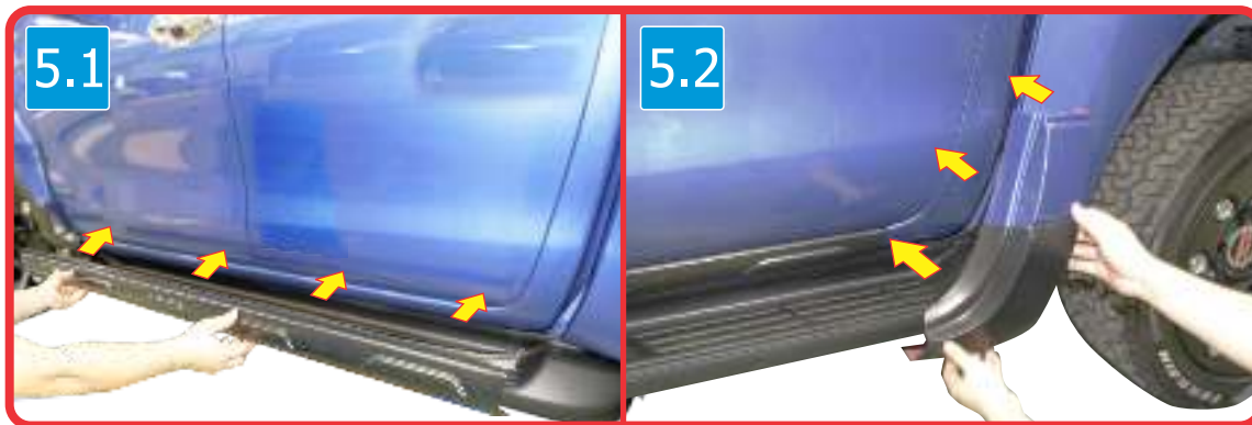
5.1 & 5.2) Install side skirt part 1 & part 2 in correct position as shown. ติดตั้งชุดสเกิร์ตข้างเข้ากับตัวรถ
