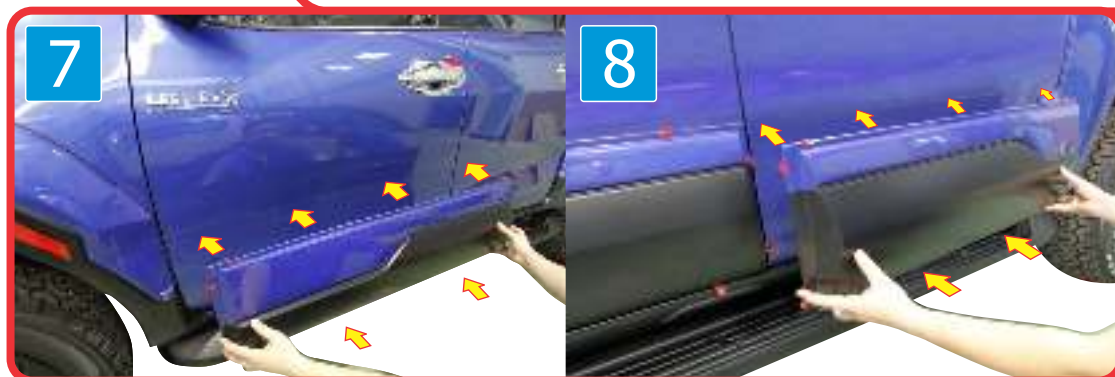
7 & 8) Install body cladding in correct position as shown. ติดตั้งกาบข้างประตู เข้ากับประตูรถ
