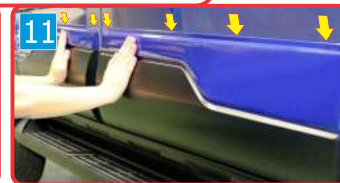
Press it firmly as shown. กดกาบข้างประตู ให้แน่นติดกับประตูรถ
