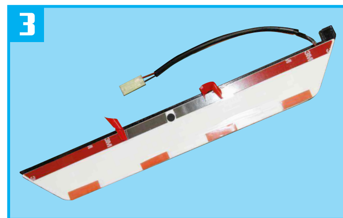
3 Peel off double sided tape on back side of led door scuff plate a bit as shown. ลอกเทปกาวชายบันไดเรืองแสงออกเพียงเล็กน้อย
