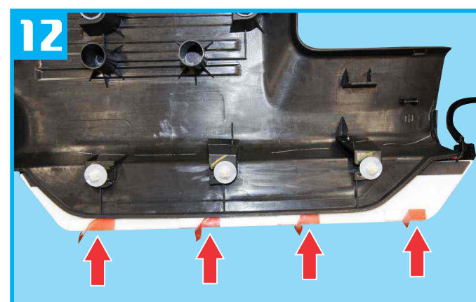
12 Peel off double sided tape on back side of led door scuff plate a bit as shown. ลอกเทปกาวชายบันไดเรืองแสงออกเพียงเล็กน้อย
