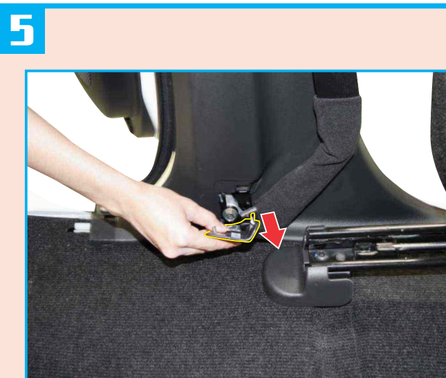
5 Remove cover pillar as shown. ถอดฝาครอบปิดเสากลางประตูออก
