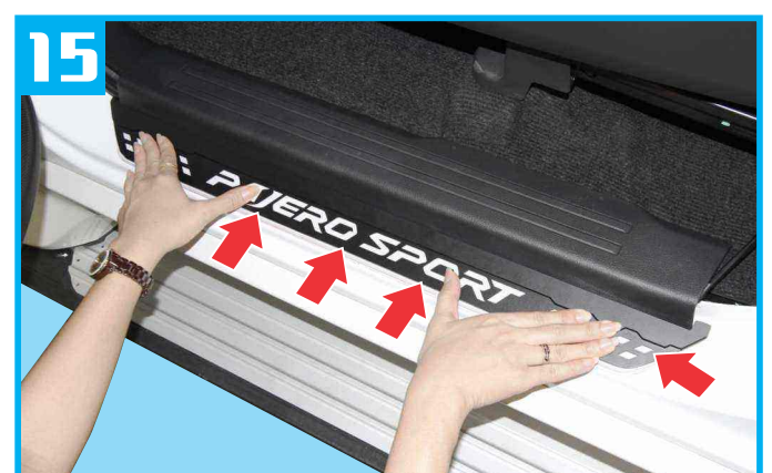
15 Press the led door scuff plate firmly to vehicle. กดชายบันไดเรืองแสงให้แน่นติดกับรถยนต์อีกครั้ง
