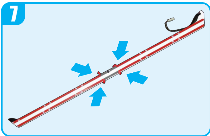
Peel off double sided tape on back side of LED door scuff plate a bit as shown. ลอกเทปกาวชายบันไดเรืองแสงออกเพียงเล็กน้อย
