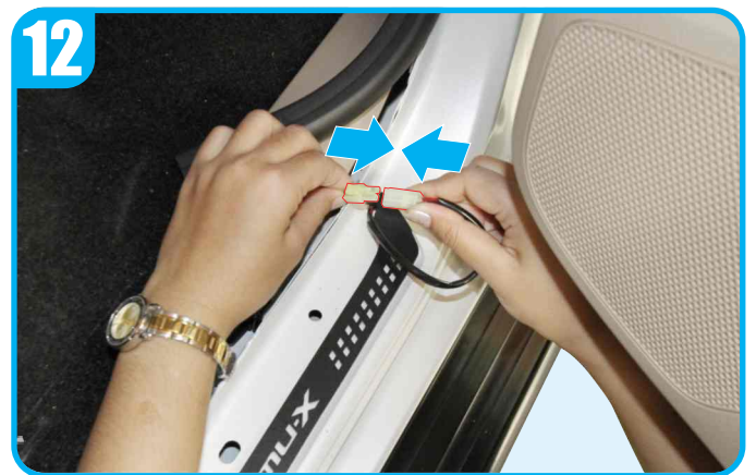
Connect the power cord into the socket of the Lamp. เชื่อมต่อขั้วปลั๊กของชายบันไดเรืองแสงเข้ากับขั้วปลั๊กของชุดสายไฟชายบันไดเรืองแสง
