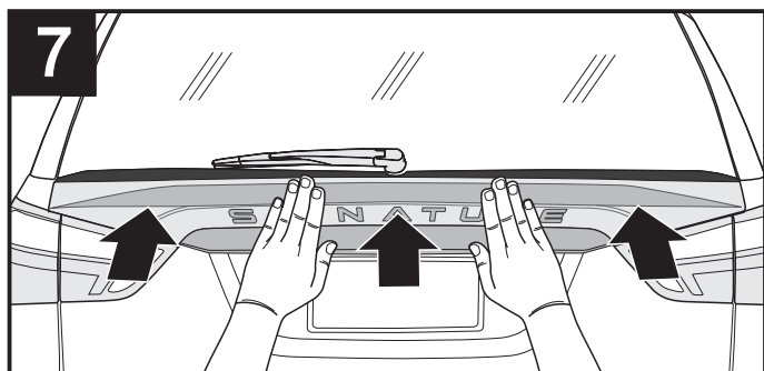
Press middle spoiler firmly. กดให้แน่นติดกับประตูท้ายของรถยนต์
