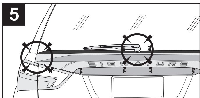
Mounting middle spoiler on correct position as shown. ติดตั้งครอบมิดเดิลสปอยเลอร์เข้ากับประตูท้ายของรถยนต์ ดังภาพ
