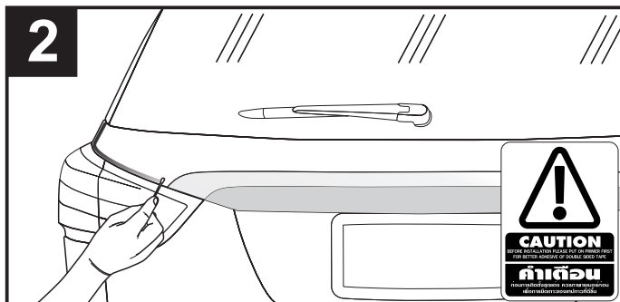
Apply Primer (provided) on position as shown. ทาน้ำยา พรายเมอร์ บริเวณที่ มิดเดิลสปอยเลอร์ ยึดติดกับตัวรถยนต์ เพื่อการยึดเกาะของเทปกาว 3M เต็มประสิทธิภาพ ดังภาพ
