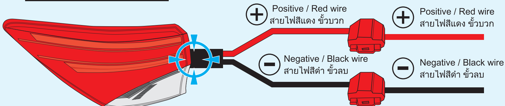
Wire of Tail lamp left hand side สายไฟไฟท้ายรถยนต์ฝั่งซ้าย
