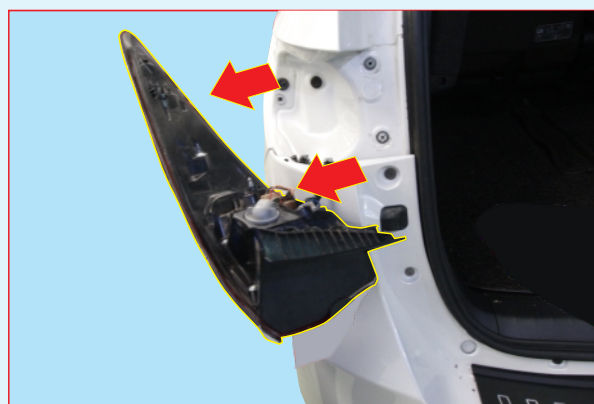
Wire of Rear bumper guard with LED สายไฟกรอบกันรอยท้ายเรืองแสง
