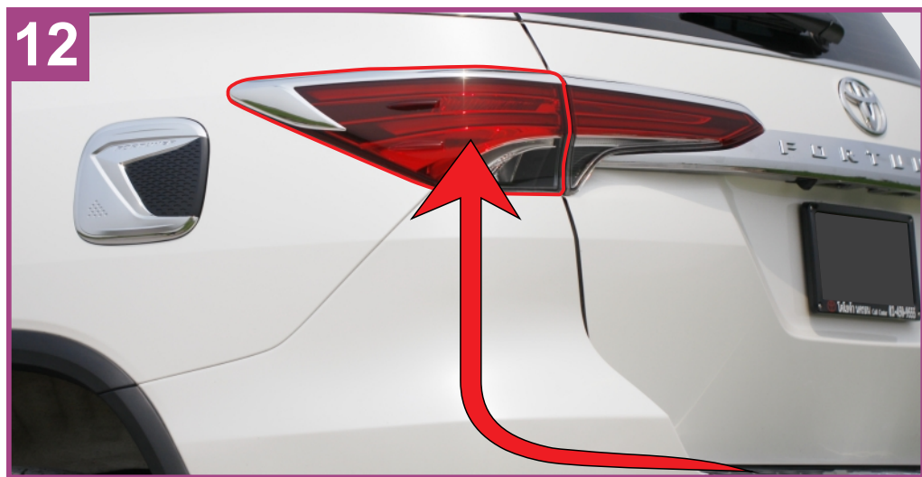
Pass wire of rear bumper guard with LED through all parts as shown. เดินสายไฟกรอบกันรอยท้ายเรืองแสงขึ้นไปไฟท้ายฝั่งซ้าย
