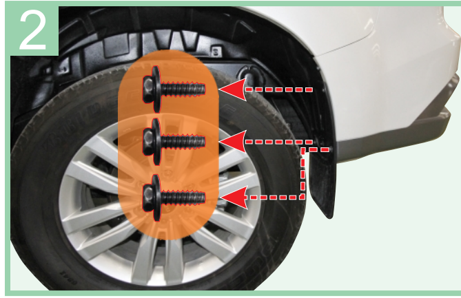
Loosen the screw on front fender flare as shown ถอดสกรูยึดซุ้มล้อ ตามภาพ
