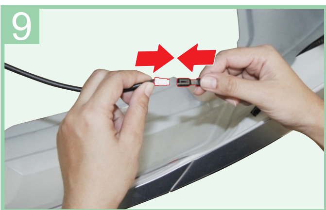
Connect LED wire of rear skirt to lamp wire as shown เชื่อมต่อสายไฟเข้ากับชุดดวงไฟ LED สเกิร์ตหลัง ตามภาพ
