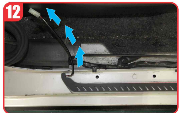
Insert scuff plate with LED wire through the interior cabin as shown. เดินสายไฟชายบันไดเรืองแสงเข้าภายในห้องโดยสาร
