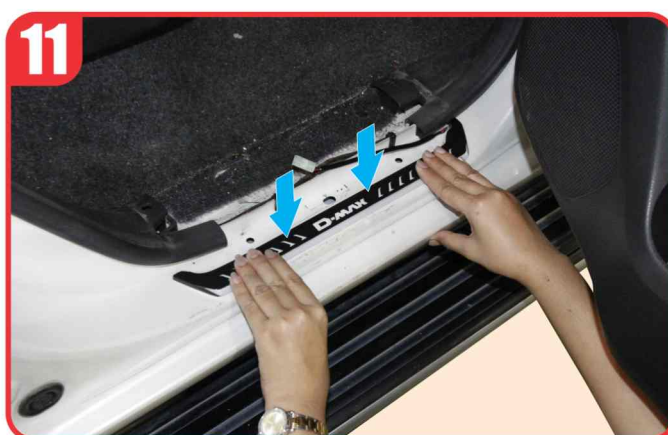
Press the LED door scuff plate firmly to vehicle. กดชายบันไดเรืองแสงให้แนบติดกับรถยนต์อีกครั้ง
