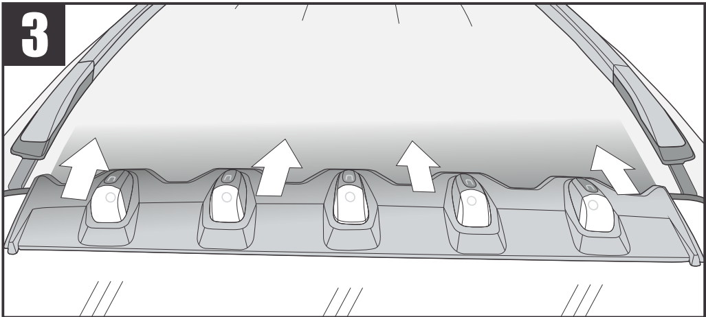
Attached LED roof kit on correct position as shown. ทาบไฟแก็ปหลังคาเข้ากับรอยนํ้า ดังภาพ
