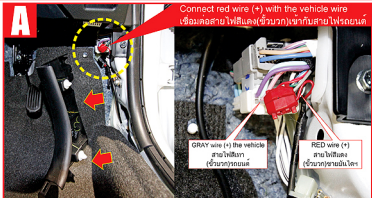
THE PROCESS OF CONNECTING SWITCH WIRE (FRONT DOOR RH) ขั้นตอนการเชื่อมต่อสายไฟสวิตช์ (ประตูหน้า ด้านขวา)
