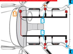
THE PROCESS OF CONNECTING SWITCH WIRE (FRONT DOOR RH) ขั้นตอนการเชื่อมต่อสายไฟสวิตช์ (ประตูหน้า ด้านขวา)
